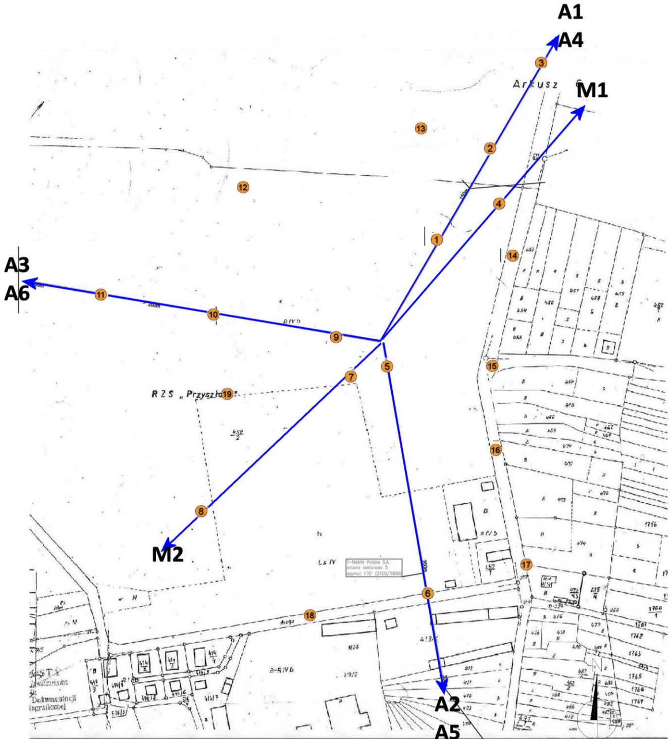
Azymuty anten
