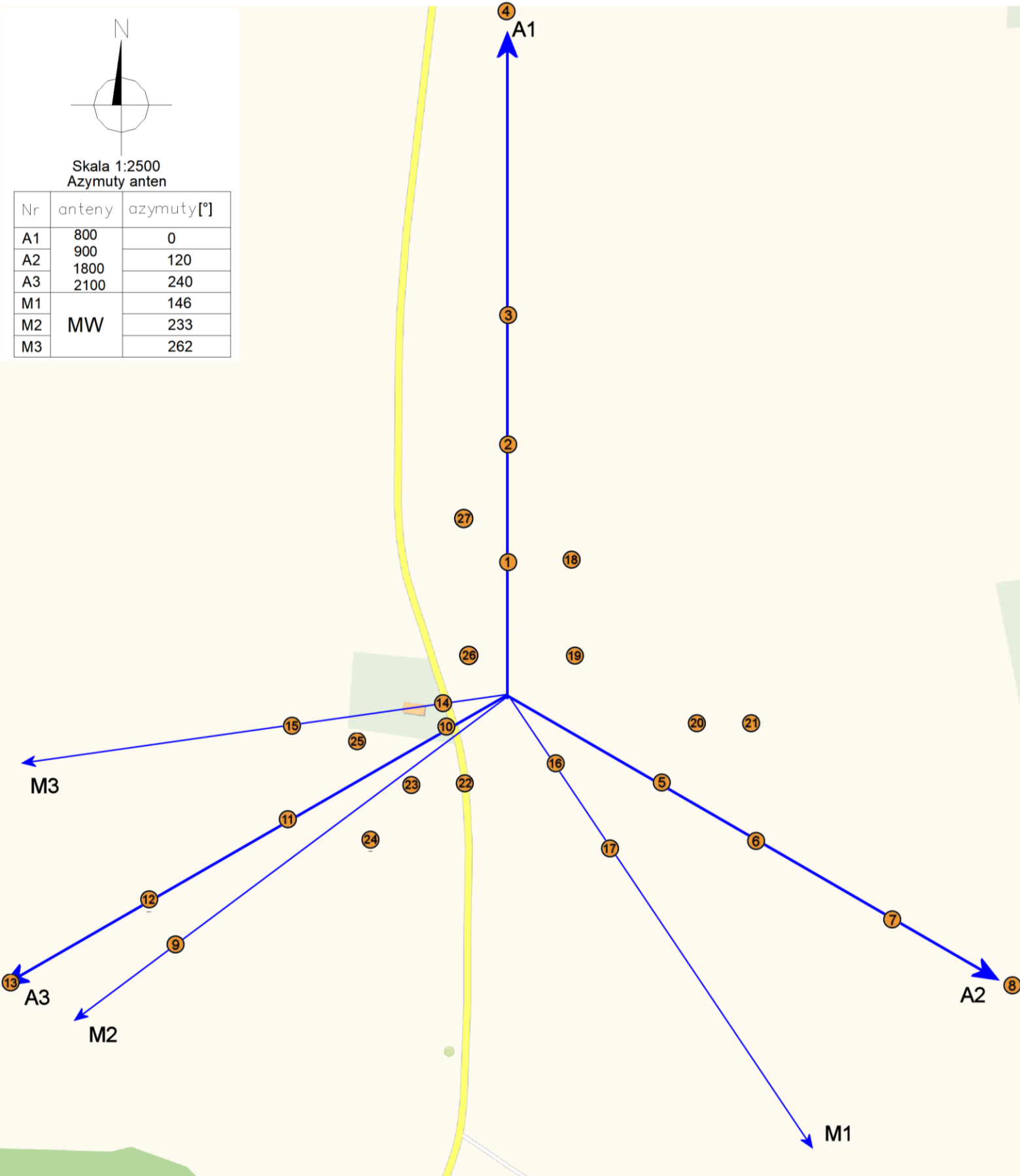
ZaŃ. nr 2: Lokalizacja anten oraz ich azymuty, lokalizacja pionów (punktów pomiarowych wokół instalacji radiokomunikacyjnej). -punkt (pion) pomiarowy.
